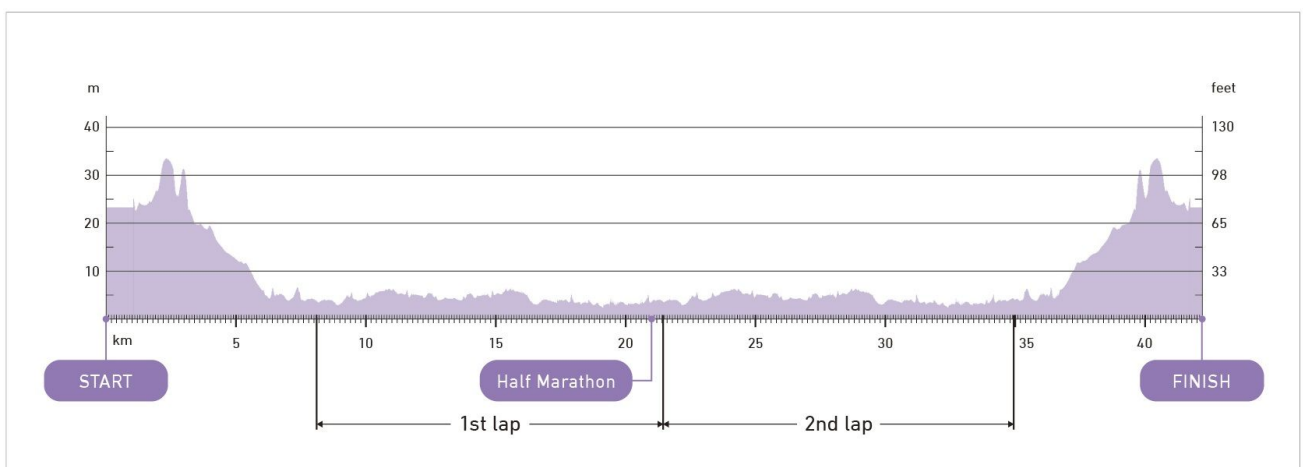
高低図
